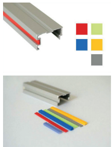
A - Profilé «H»
