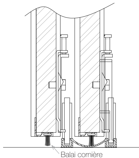
B - Balai cornière
