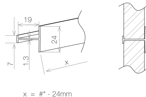
D - Profilé «H»
